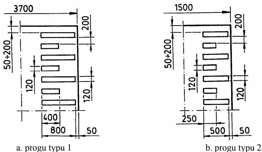
Rys. 2. Oznakowanie poziome
